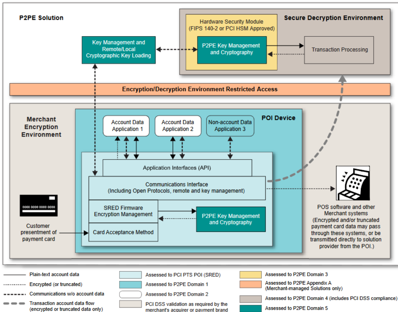
Fig.7: architettura tipica P2PE (rif. PCI P2PE ver 3.1)
