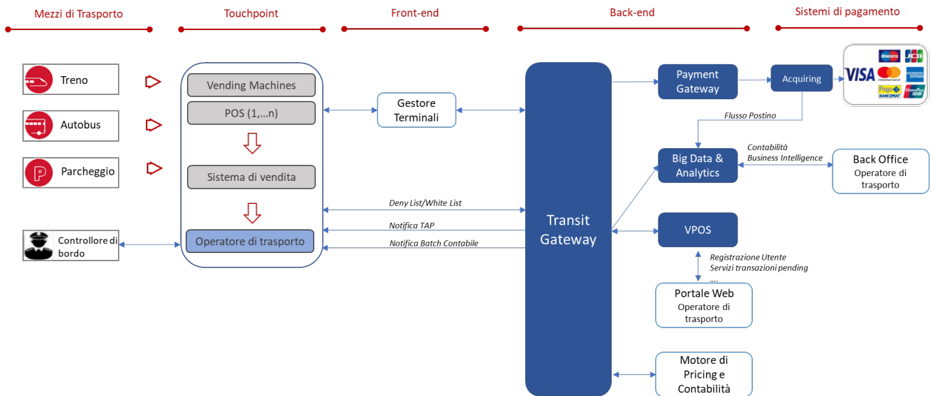
Fig.9: Esempio di schema architetturale Transit
